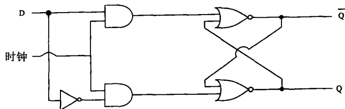
图A-12 一个D触发器
