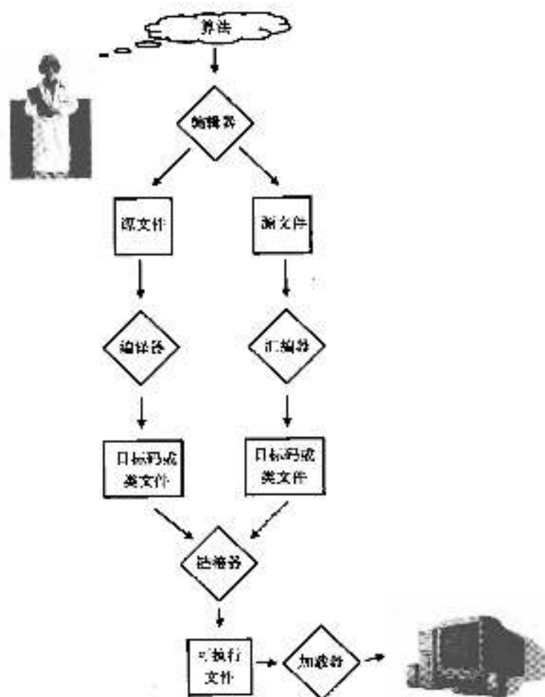
图1-18 编程过程
