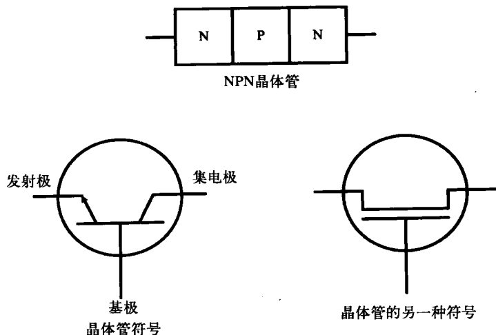
图1-6 晶体管
