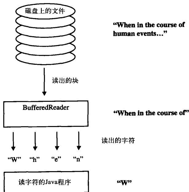
图10-18 使用BufferedReader从磁盘读入一个文件
