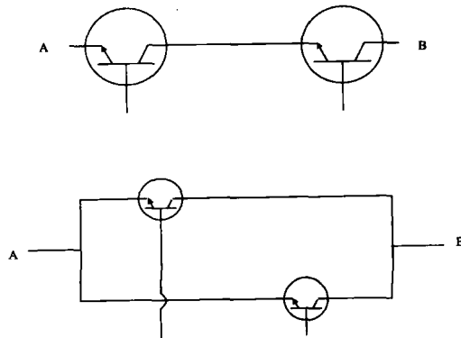
图A-2 串联（上图）和并联（下图）的晶体管
