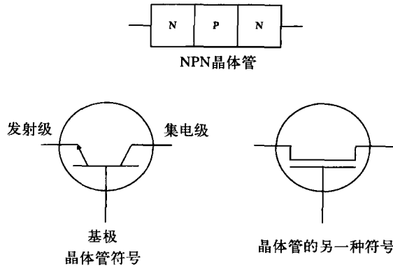
图A-1 晶体管和符号的样例
