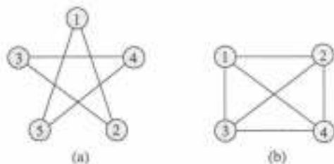
图 0-5 图的例子
