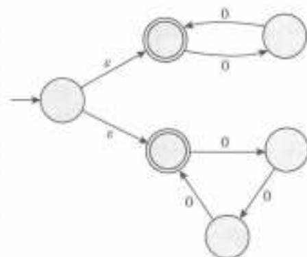
图 1-19 NFA N_3
