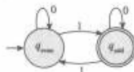
图 1-12 增加起始状态和接受状态
