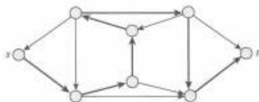
图 7-3 哈密顿路径经过每个结点恰好一次
