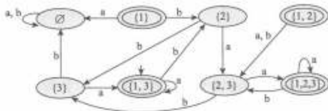
图 1-22 与 NFA N_1 等价的 DFA D
