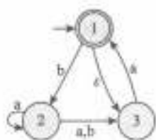
图 1-21 NFA N_1
