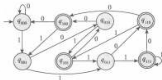
图 1-18 一台识别 A 的 DFA
