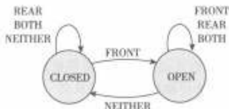
图 1-2 自动门控制器的状态图
