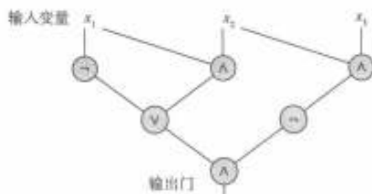
图 9-3 布尔电路的例子
