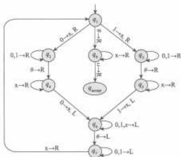
图 3-5 图灵机 M_3 的状态图
