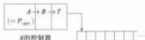
图 6-2 R 的图示
