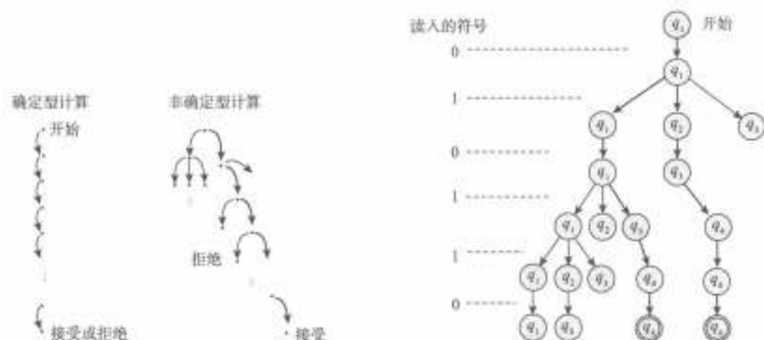
图 1-15 有一个接受分支的确定型计算和非确定型计算
