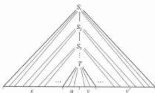
图 2-18 派生 xuvy' 的语法树
