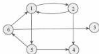
图 0-9 一个有向图
