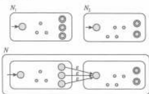
图 1-25 识别 A_1 \cdot A_2 的 N 的构造
