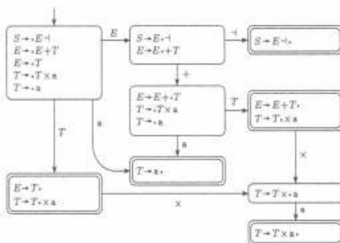
图 2-20 一个失败的 DK -测试例子
