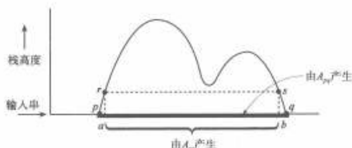
图 2-14 对应规则 A_{pq} \rightarrow aA_n b 的 PDA 计算
