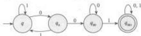
图 1-13 接受含有 001 的字符串
