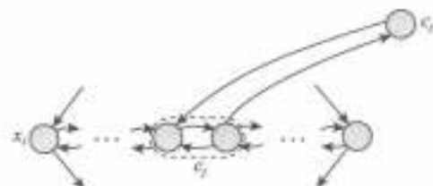
图 7-17 当子句 c_j 包含 \bar{x}_i 时添加的边
