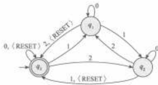
图 1-9 有穷自动机 M_5
