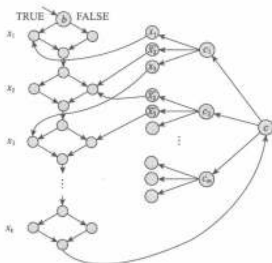
图 8-5 模拟公式博弈的地理学游戏的全部结构，其中 \phi = \exists x_1 \forall x_2 \dots \exists x_n [(x_1 \vee \bar{x}_2 \vee x_3) \wedge (\bar{x}_2 \vee \bar{x}_1 \vee \dots) \wedge \dots \wedge ( )]
