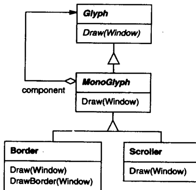
图2-7 MonoGlyph类关系
