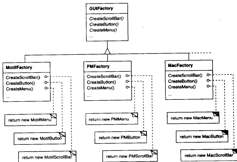
图2-9 GUIFactory类层次
