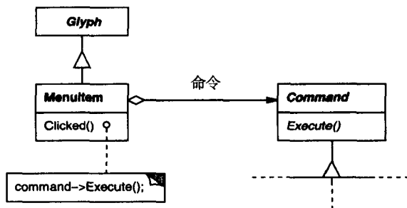
图2-12 MenuItem-Command关系
