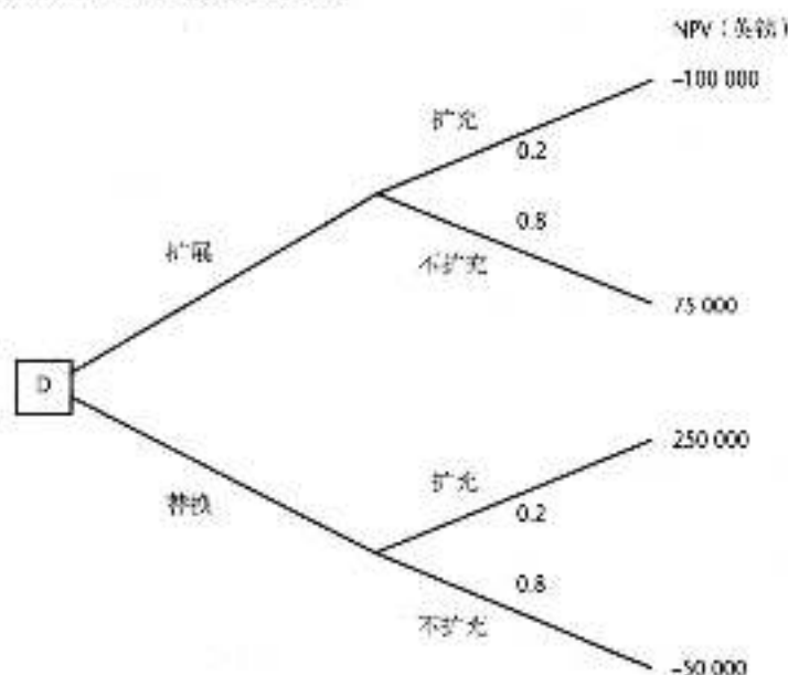
图2-2 决策树
