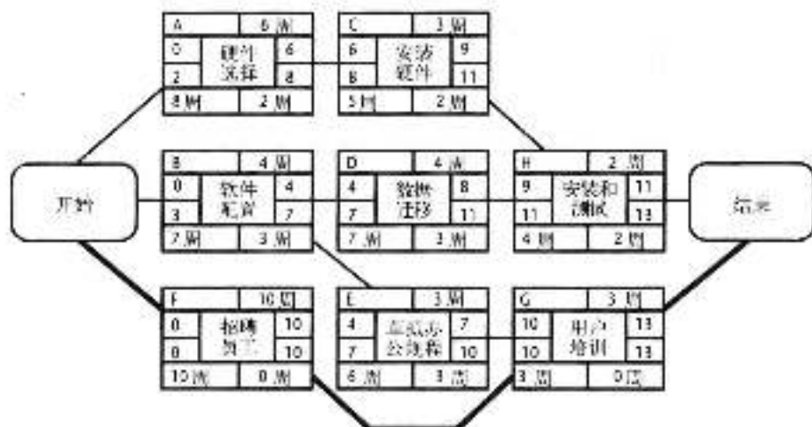
图6-17 关键路径
