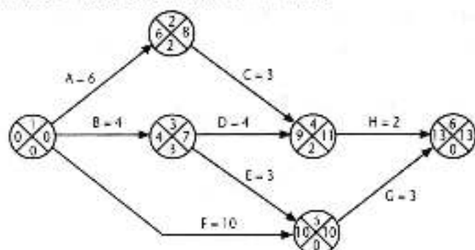
图6-29 关键路径
