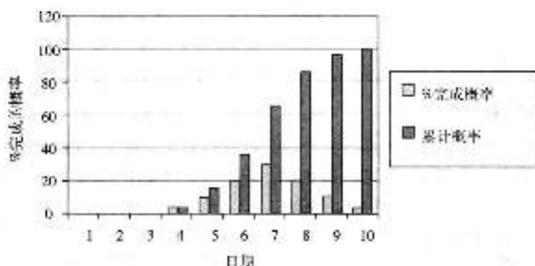
图7.3 概率图
