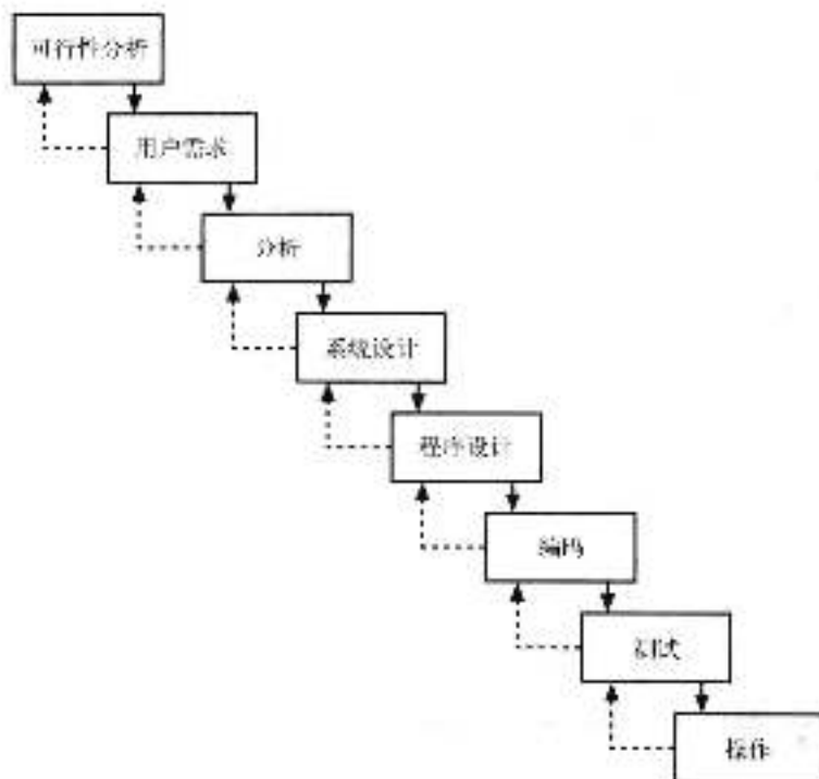
图4-2 瀑布模型
