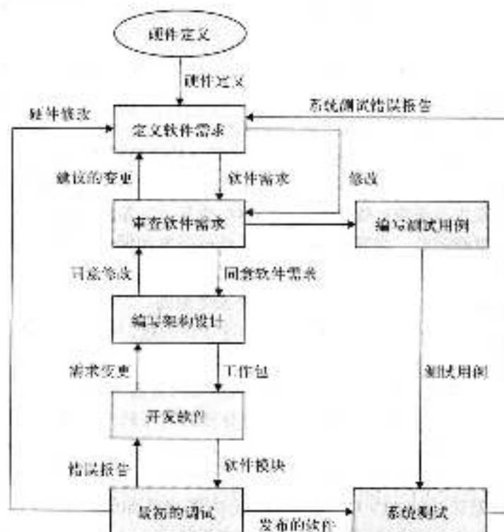
图13-4 流程图
