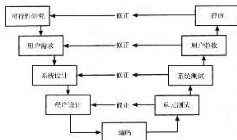
图13-5 V模型
