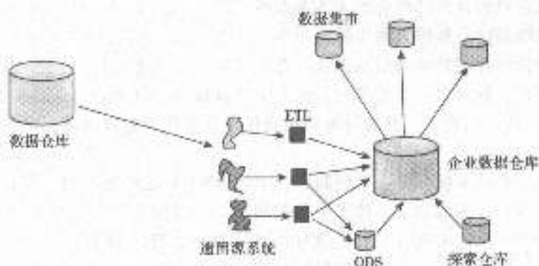
图 1-5 数据仓库很快就被演变为一个被称为企业信息工厂的成熟构架
