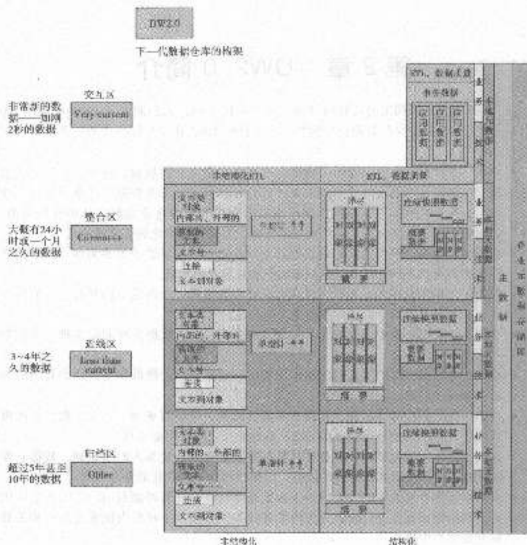
图 2-1 DW2.0 的数据结构
