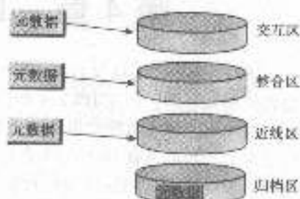
图4-1 元数据及 DW2.0 环境
